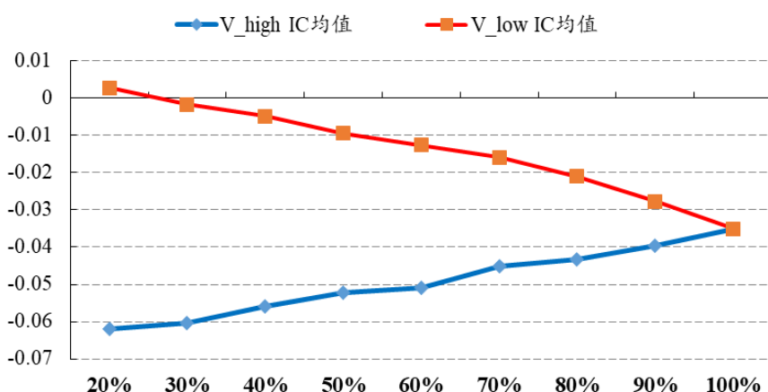
图8：不同 \lambda 值下高价振幅因子和低价振幅因子 IC 均值差距单调变化
